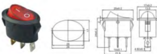
A-TOP1-9-101N ON-OFF
