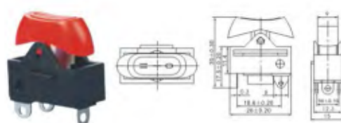
A-TOP1-122-1 OFF-ON-ON
