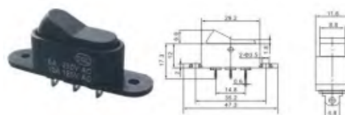
A-TOP1-13-102 ON-ON
