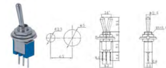
BTS-102-A2 ON-ON SPDT 3P
